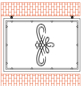
DISEGNO 2
