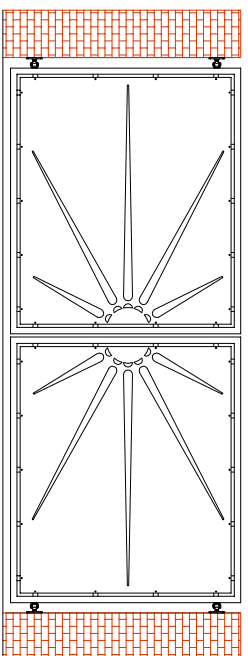
DISEGNO 13-bis SOLO FINO A LUNGH. 3500
